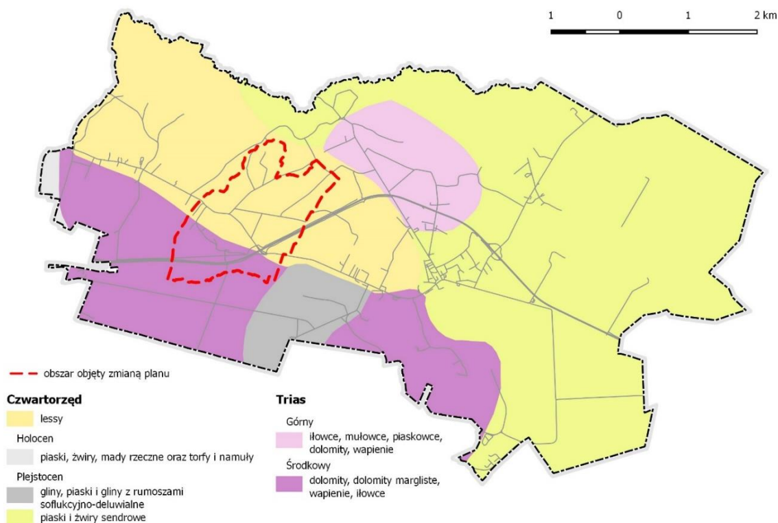
Ryc. 4. Budowa geologiczna Gminy Bolesław
