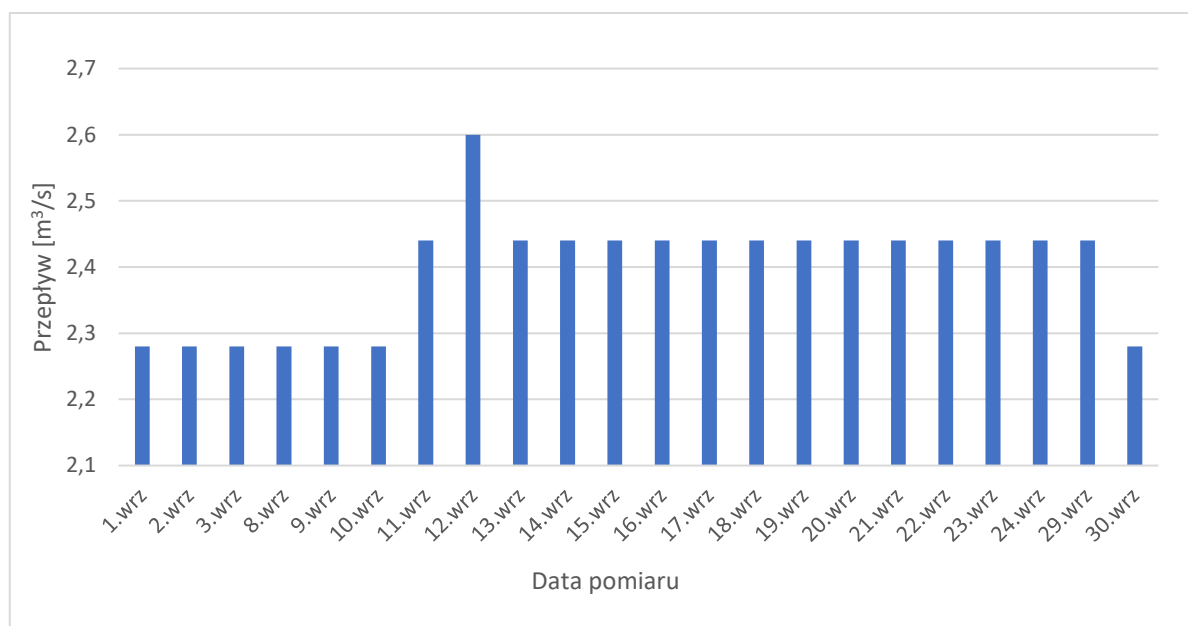
Ryc. 1. Wyniki pomiarów przepływów na rzece Biała Przemsza na stacji hydrologicznej w Sławkowie we wrześniu 2026 r. (źródło: IMGW).
