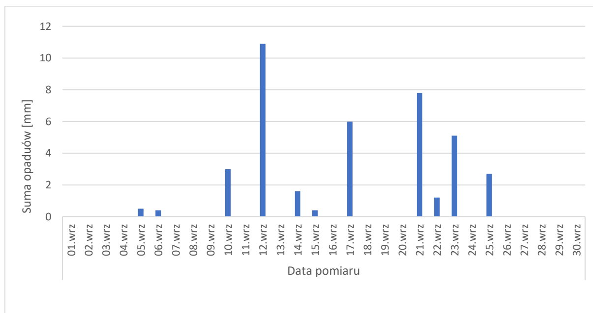
Ryc. 2. Suma opadów dobowych na stacji meteorologicznej IMGW w Troksie we wrześniu 2026 r. (źródło: IMGW).
