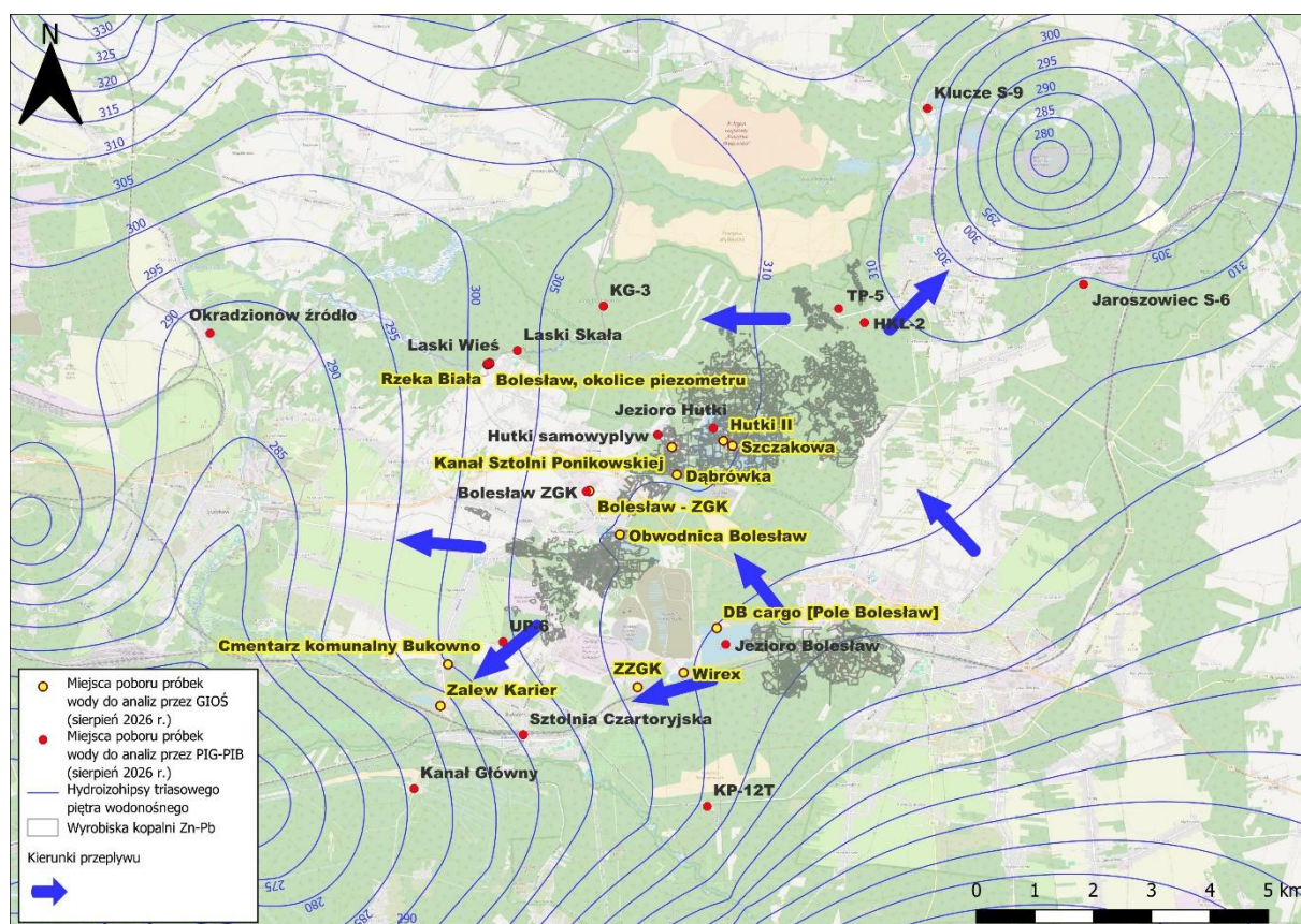
Ryc. 12. Lokalizacja miejsc poboru próbek wody do analiz przez GIOŚ i PIG-PIB w centrum regionu olkuskiego (opracowanie własne PIG-PIB).
