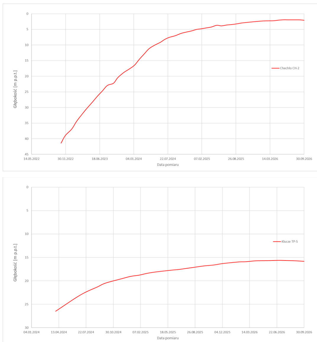
Ryc. 9. Wykresy zmian położenia zwierciadła wody w wybranych punktach monitoringowych (opracowanie własne PIG-PIB).
