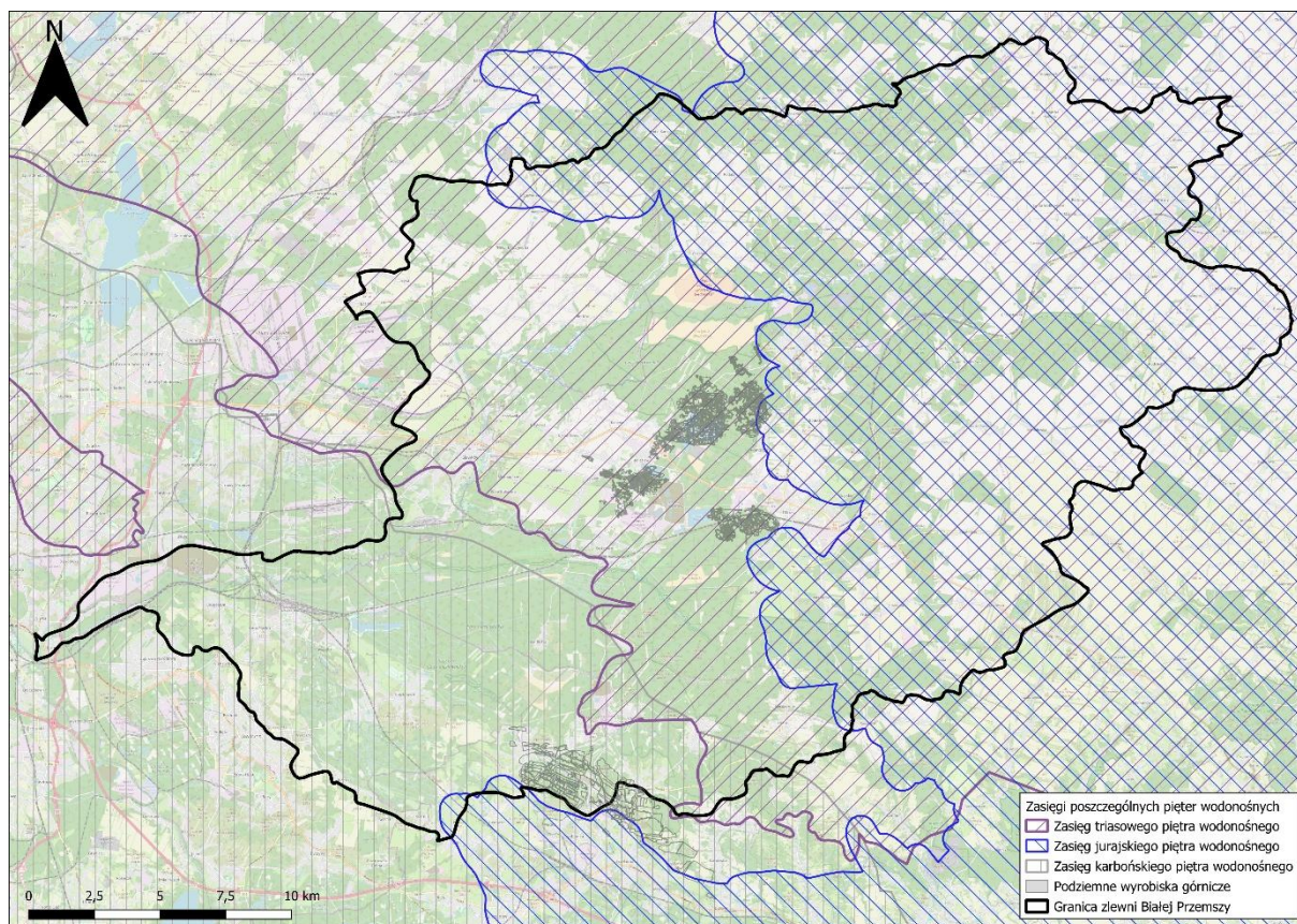
Ryc. 6. Zasięg występowania głównych pięter wodonośnych. (na podstawie MGP 1:500 000, PIG-PIB 2024 r., opracowanie własne PIG-PIB).
