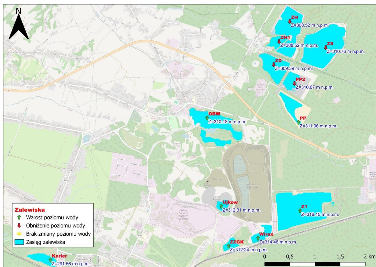
Ryc. 3. Mapa zalewisk w rejonie olkuskim (na podstawie pomiarów ZGH „Bolesław”) stan na 23.09.2026 r. Strzałkami oznaczono zmianę położenia zwierciadła wody w stosunku do poziomu raportowane w poprzednim Raporcie 8 (opracowanie własne PIG-PIB).
