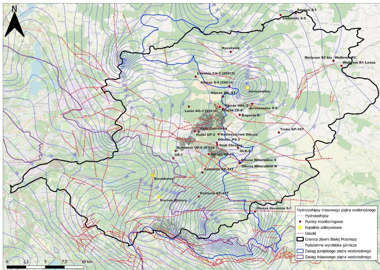
Ryc. 7. Rozkład rzędnych zwierciadła wód podziemnych w triasowym (w zasięgu występowania) i czwartorzędowym pięttrze wodonośnym, stan na wrzesień 2026 r (opracowanie własne PIG-PIB).
