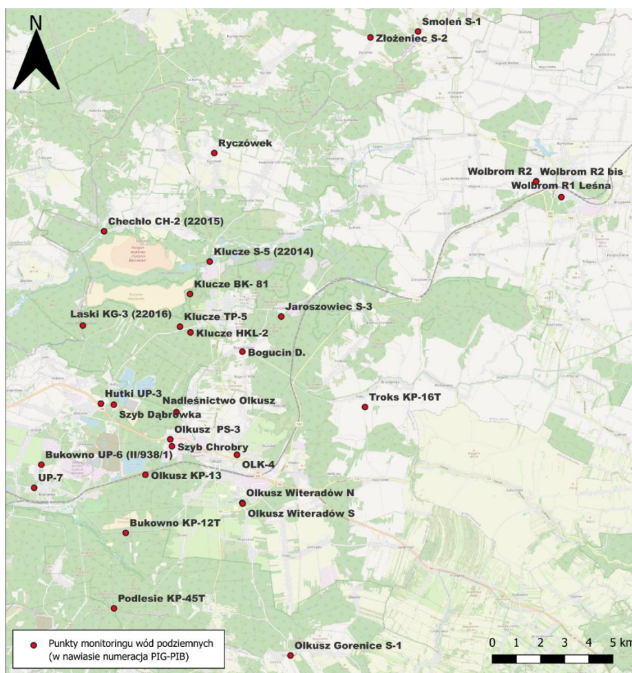
Ryc. 5. Lokalizacja punktów monitoringu wód podziemnych w rejonie olkuskim (opracowanie własne PIG-PIB).
