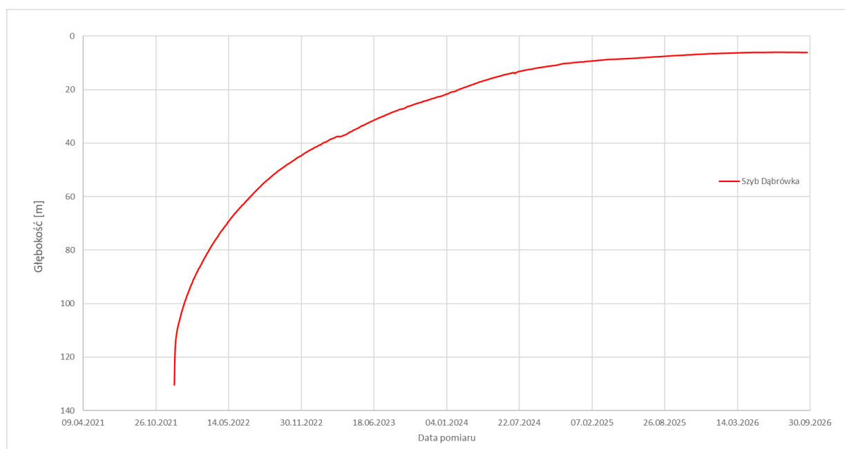
Ryc. 10. Wykresy zmian położenia zwierciadła wody w szybie Dąbrówka oraz Chrobry (opracowanie własne PIG-PIB).
