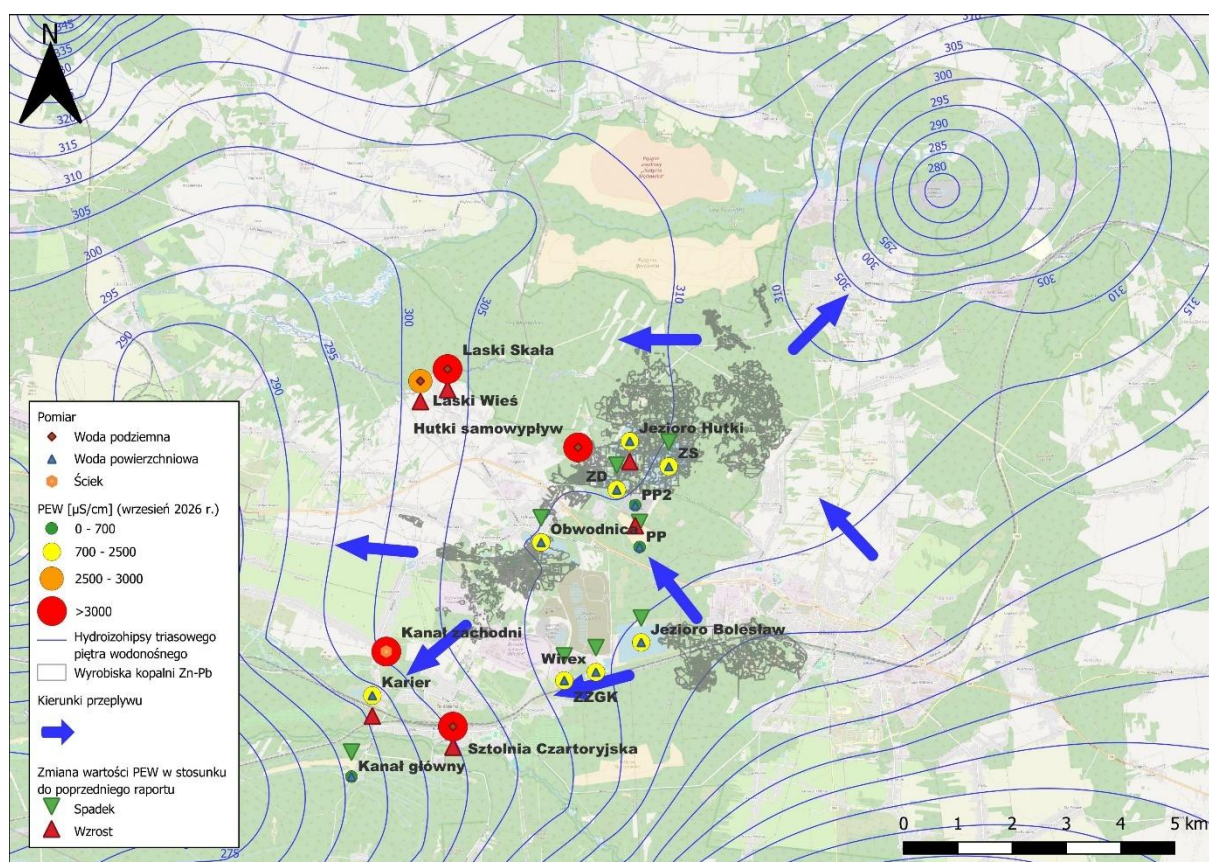
Ryc. 11. Mapa rozkładu przewodności elektrolitycznej właściwej (PEW) w obszarze badań (wrzesień 2026 r.) (opracowanie własne PIG-PIB).
