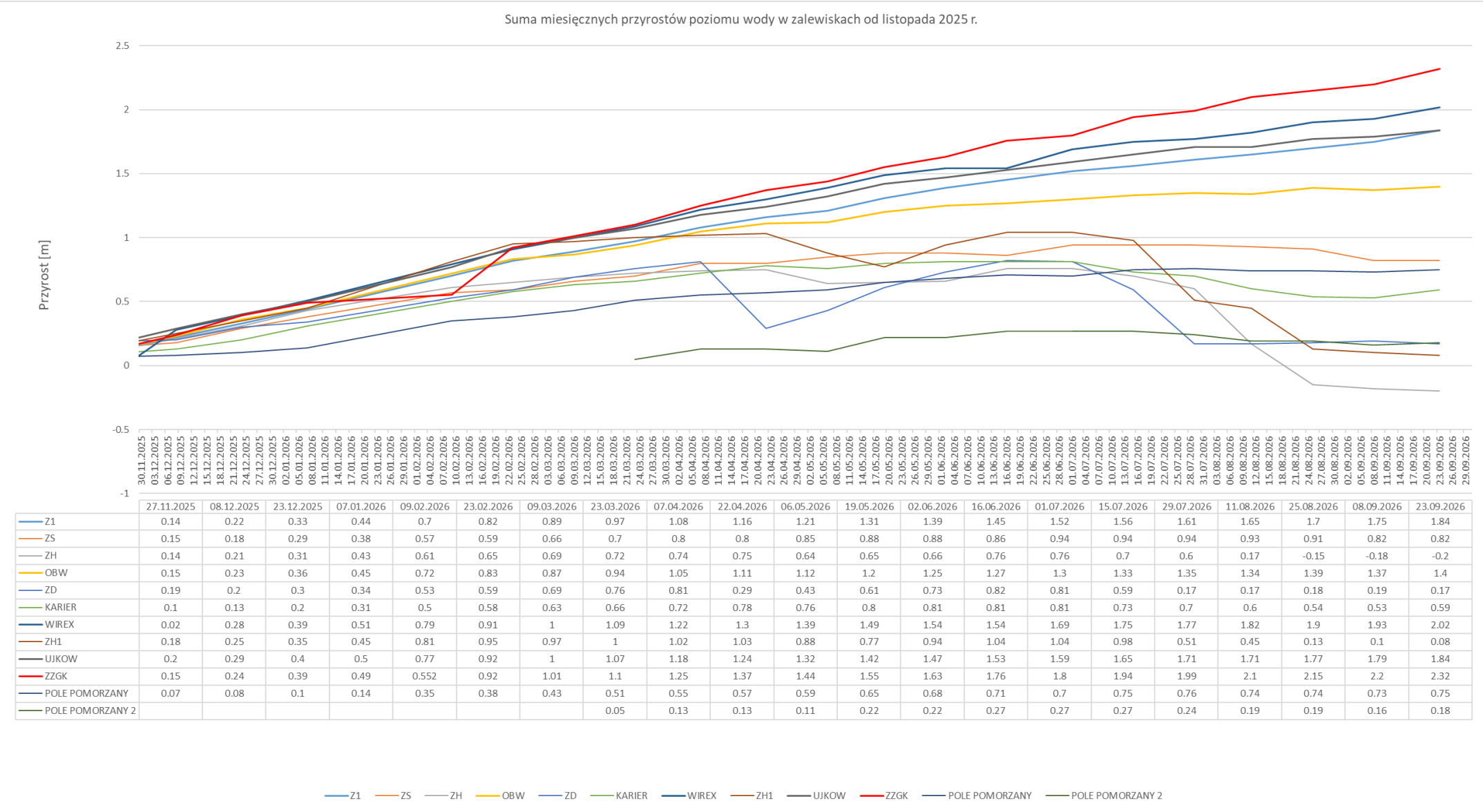
Ryc. 4. Przyrost poziomu wody w zalewiskach od listopada 2025 r do września 2026 r. (lokalizacja zalewisk przedstawiona na Ryc. 3) (opracowanie własne PIG-PIB).
