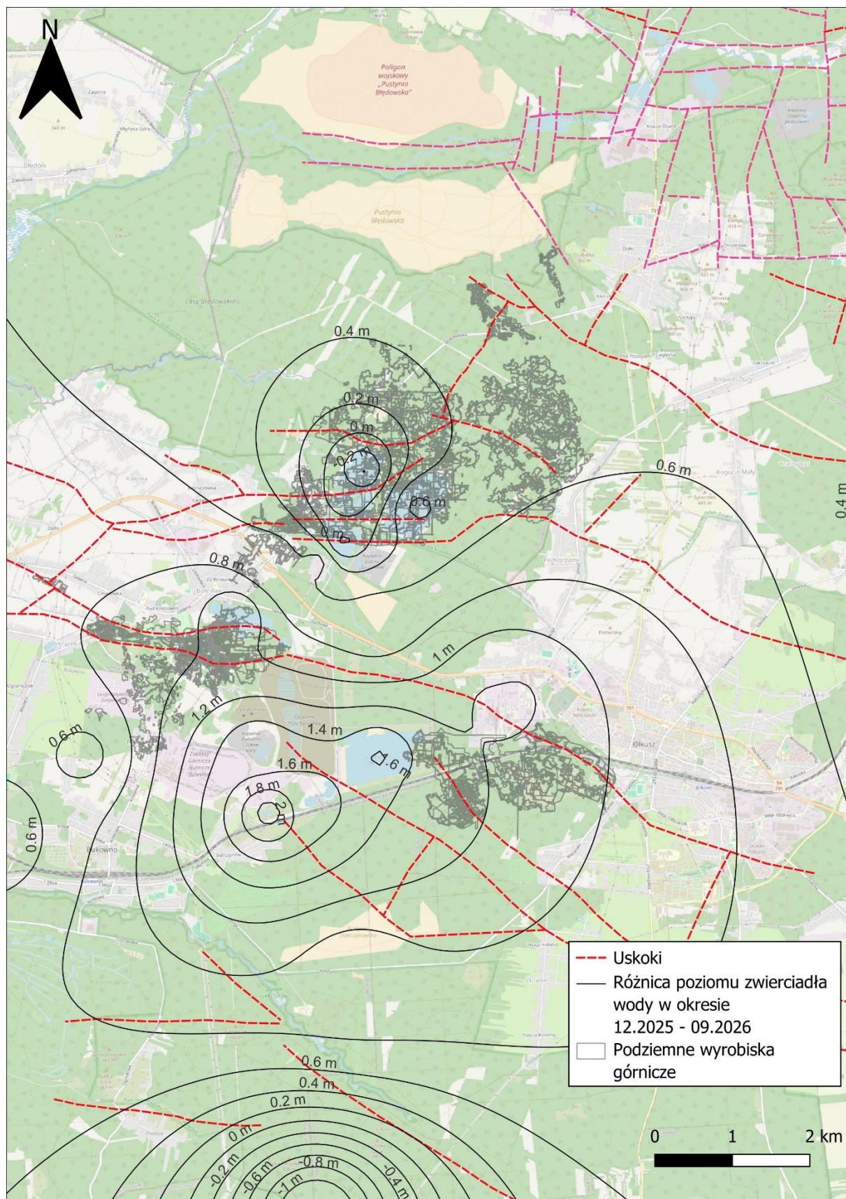
Ryc. 8. Zmiana położenia zwierciadła wody w piętrze triasowym w okresie od grudnia 2025 r. do września 2026 r (opracowanie własne PIG-PIB).
